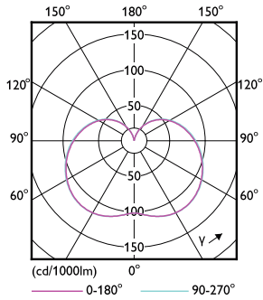
LEDTForce 65W Tshape E40 865
