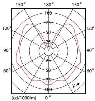
CLA LEDbulb 14W E27 820 CL A60
